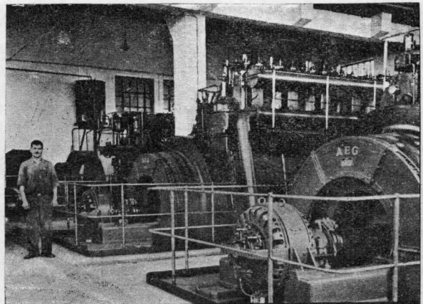
Εἰκ. 3. Τὸ μηχανοστάσιον τοῦ Ἔργοστασίου Λαδοπούλου.
