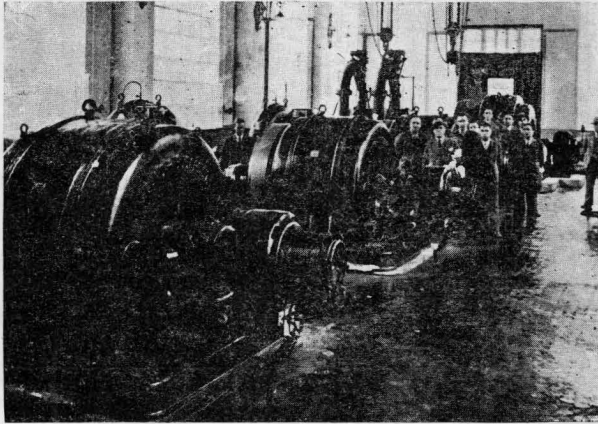
Εἰκ. 4. Οἱ τέσσαρες ὑδροστρόβιλοι τοῦ Ἵδρηνλεκτρικοῦ ἔργου αἰσίου Α.Ε. «Γλαῦκος».
