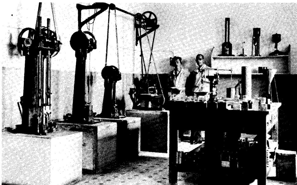
Τὸ ἐργοστάσιον Τσιμέντων «Γιτάν» εἰς τὴν Ἐλευσίνα.
