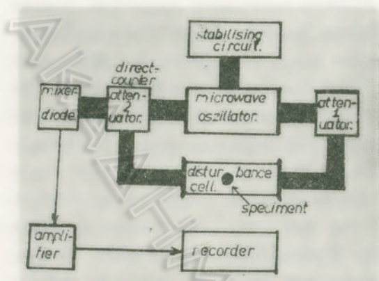
Fig. 1. Blockdiagramm der benutzten Mikrowellenanordnung.
