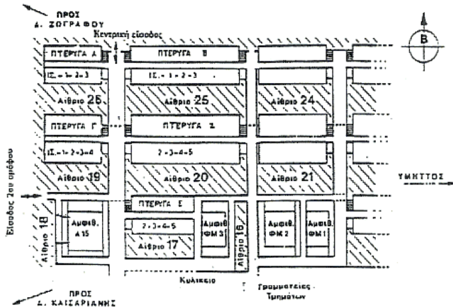
Συνοπτικό αρχιτεκτονικό σχεδιάγραμμα του βορειοδυτικού τμήματος του κτηριακού συγκροτήματος των Θετικών Επιστημών, όπου στεγάζονται τα εργαστήρια και οι χώροι διδασκαλίας του Τμήματος Χημείας.
